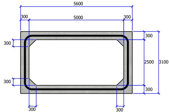
Vooraanzicht
