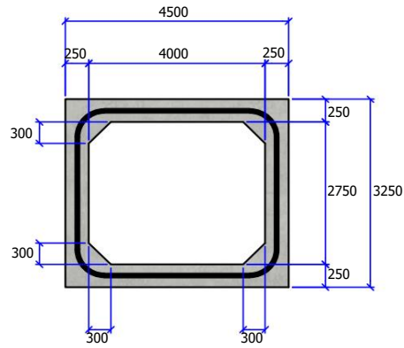
Vooraanzicht
