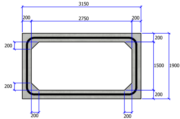
Vooraanzicht
