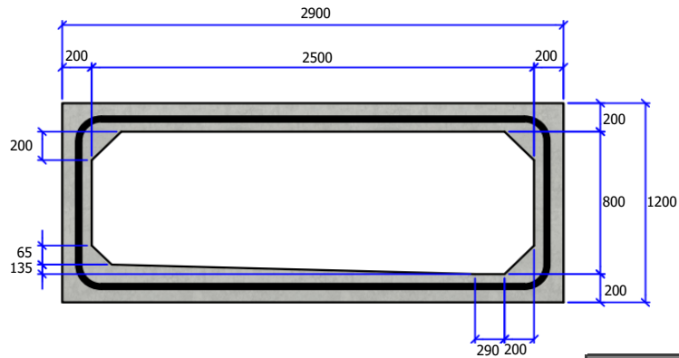
Vooraanzicht
