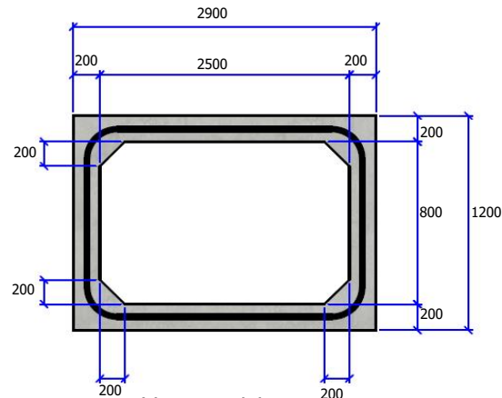
Vooraanzicht
