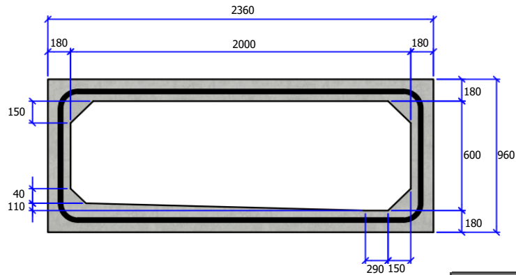
Vooraanzicht
