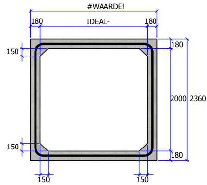
Vooraanzicht
